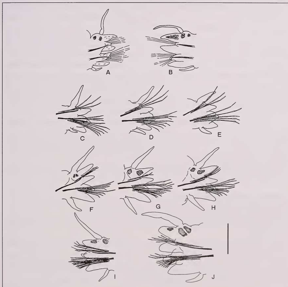
Figura 1. Ceratonereis (Composetia) costae .- Evolución de la forma de los parápodos en juveniles y adultos. A: Parápodo de Ceratonereis costae según FAUVEL [4]; B: parápodo de C. hircinicola según FAUVEL [4]; C-E: tercer, cuarto y quinto setífero de C. costae juvenil fase temprana; F-H: tercer, cuarto y quinto setífero de C. costae juvenil fase tardía; I: tercer parápodo de C. costae adulto; J: tercer parápodo de C. costae adulto.
